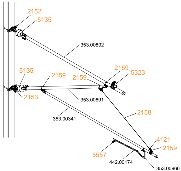
Umgelenkte Spurhaltung
