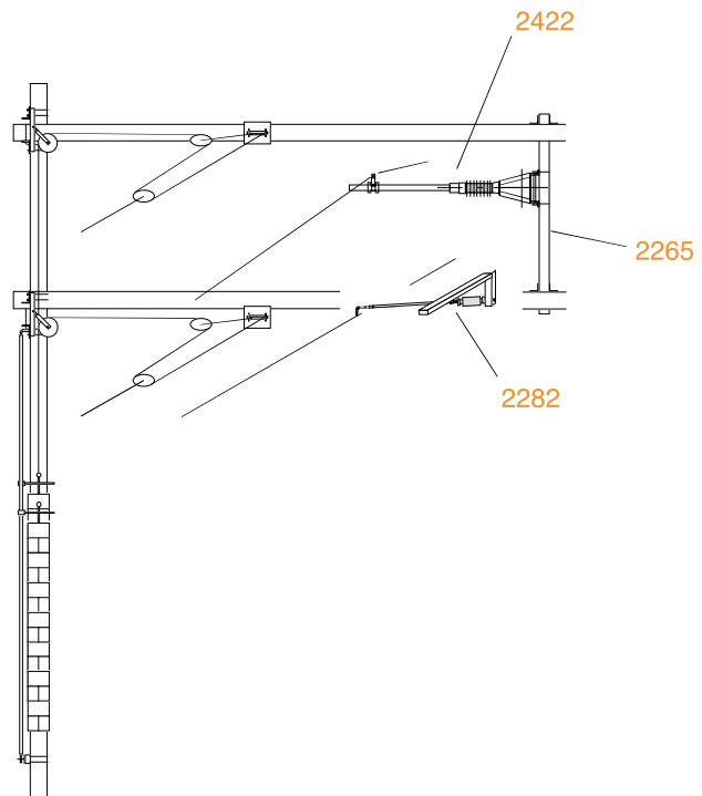
Amarrage mobil pour fil de contact et câble porteur
