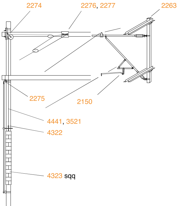
Amarrage mobil pour câble porteur
