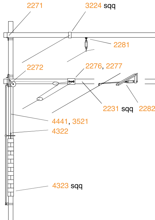
Amarrage mobil pour fil de contact et ferme pour câble porteur
