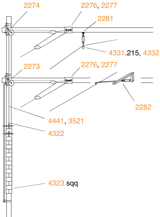
Amarrage mobil pour fil de contact et câble porteur
