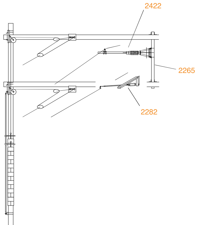
Fahrdraht und Tragseil beweglich abgespannt
