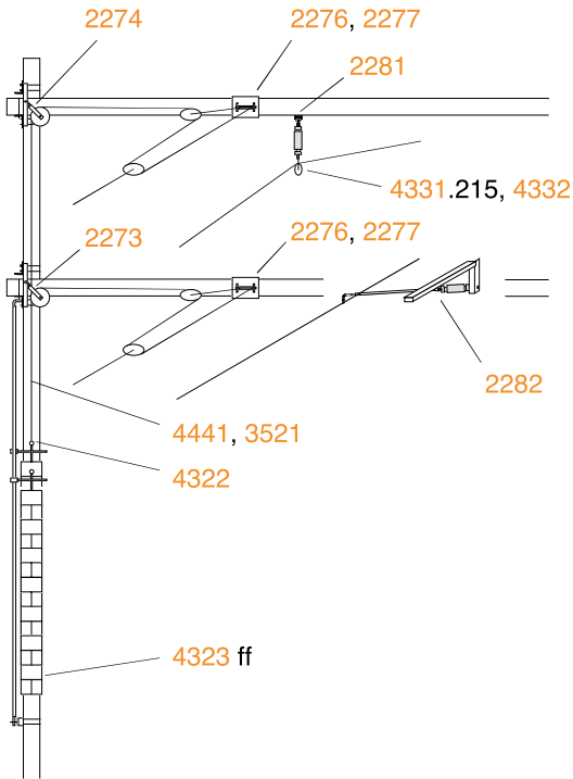
Fahrdraht und Tragseil beweglich abgespannt
