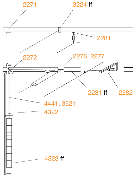
Fahrdraht beweglich, Tragseil fest abgespannt
