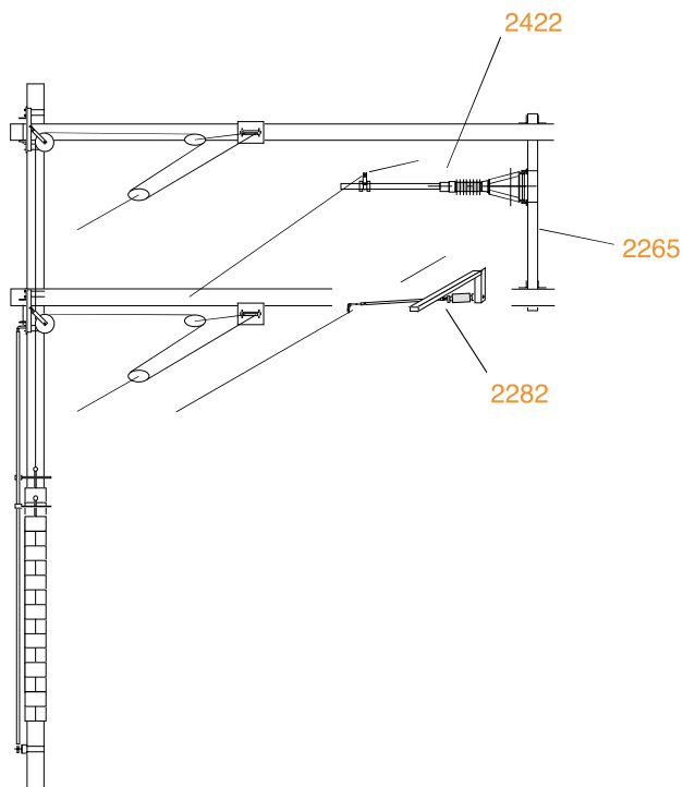
Fahrdraht und Tragseil beweglich abgespannt
