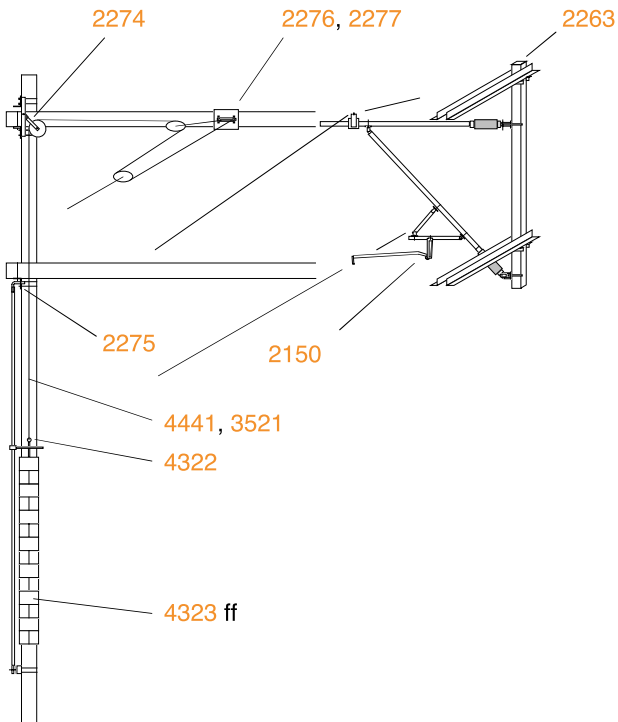
Tragseil beweglich abgespannt
