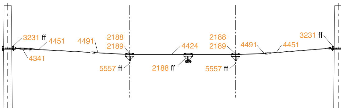
Querspanner gerade
