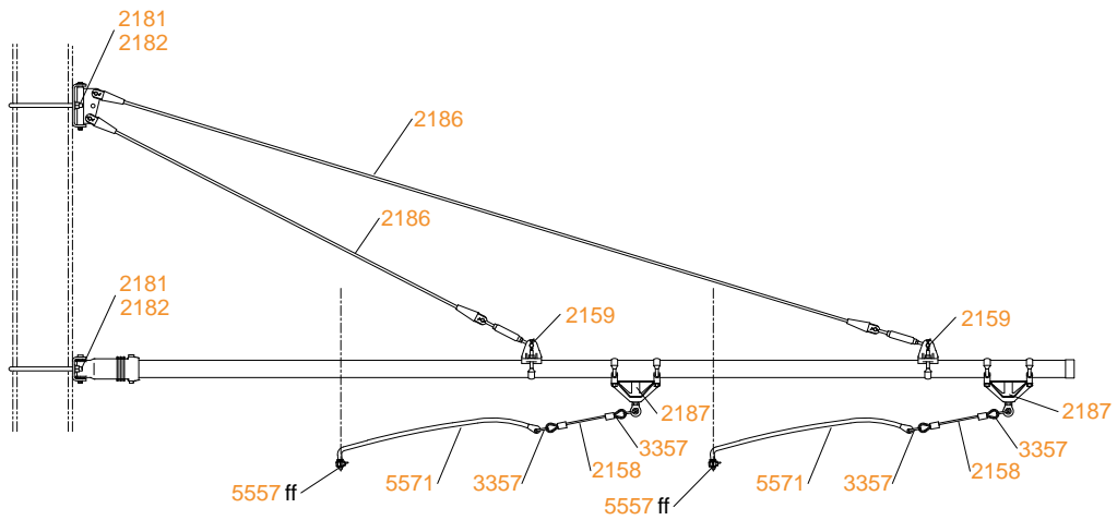
Rohrausleger über zwei Gleise mit Flachlagespurhalter
