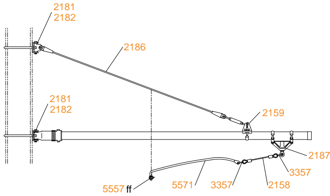
Rohrausleger über zwei Gleise mit Flachlagespurhalter
